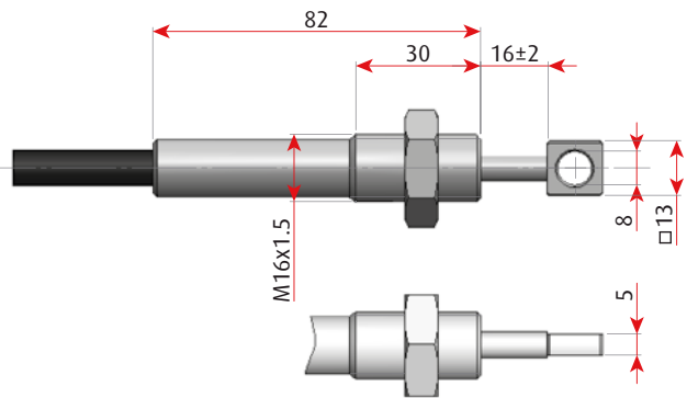
▲ Cable type 07E, code 0075921*mmmmm
