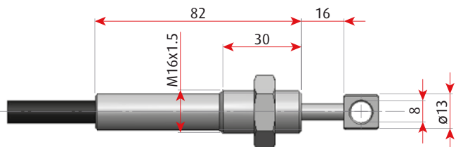
◀ Cable type 07E, code 0076200*mmmm
